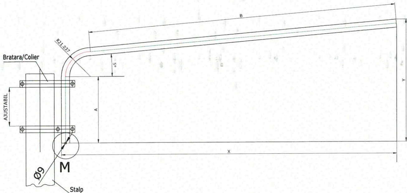
M Scara 1:2
