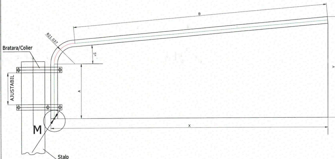
M Scara 1:2
